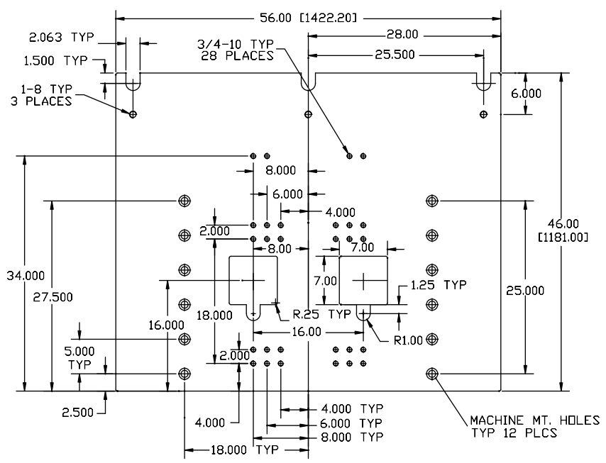
PLATEN, 3.00" REAR
